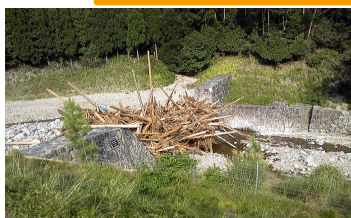
写真⑧ 土砂・立木の捕捉状況 (宍粟市 谷川砂防えん堤)
