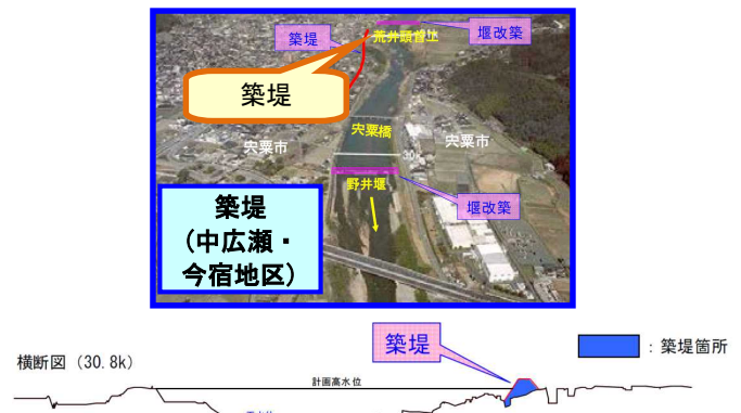
築堤による対策の一例
