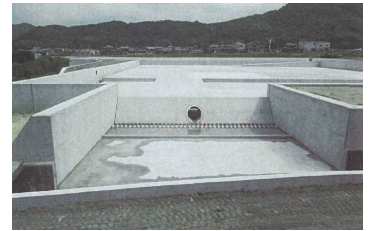
写真① 調整池の事例 (たつの市龍野町)
