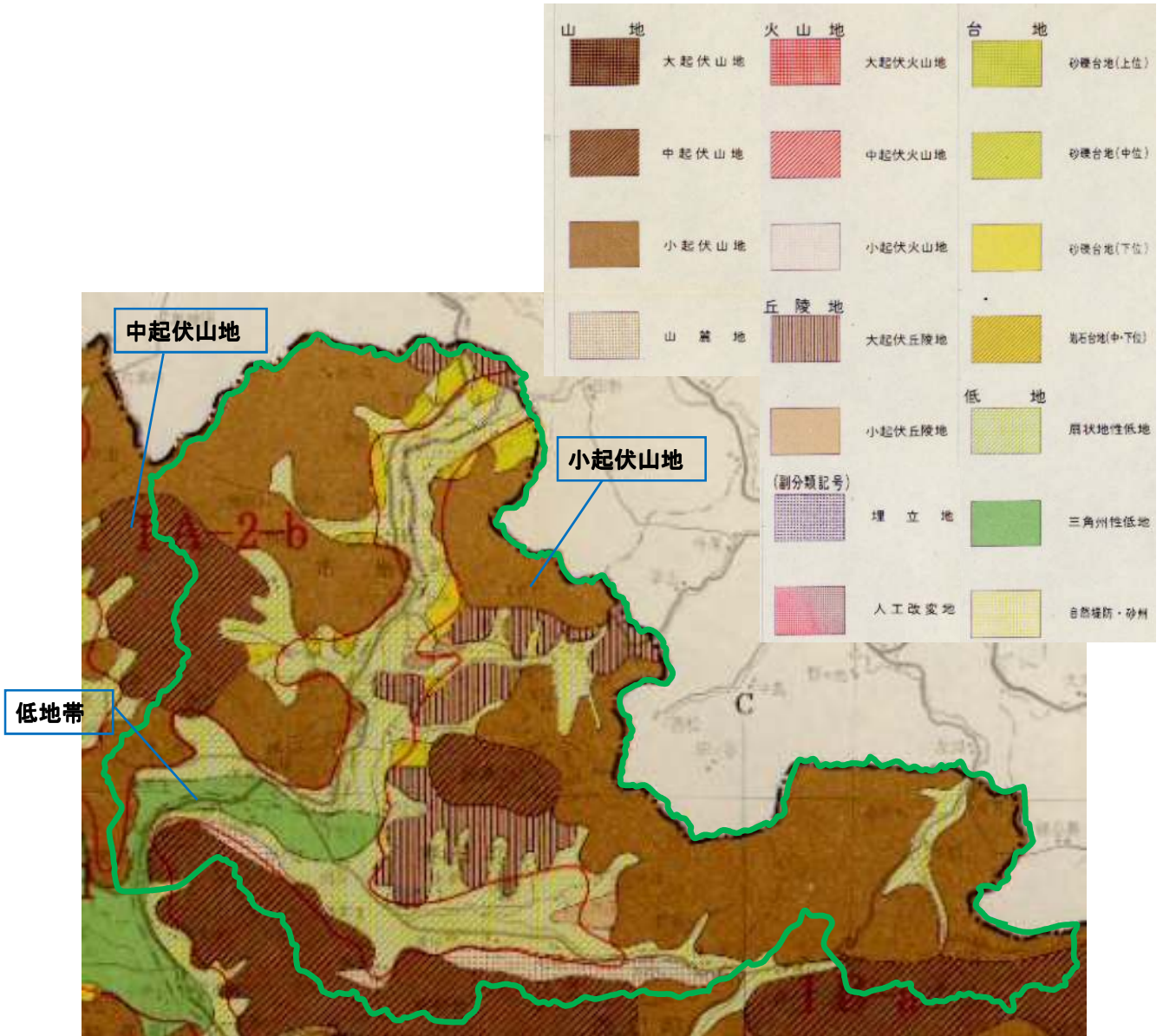
地形分類図
