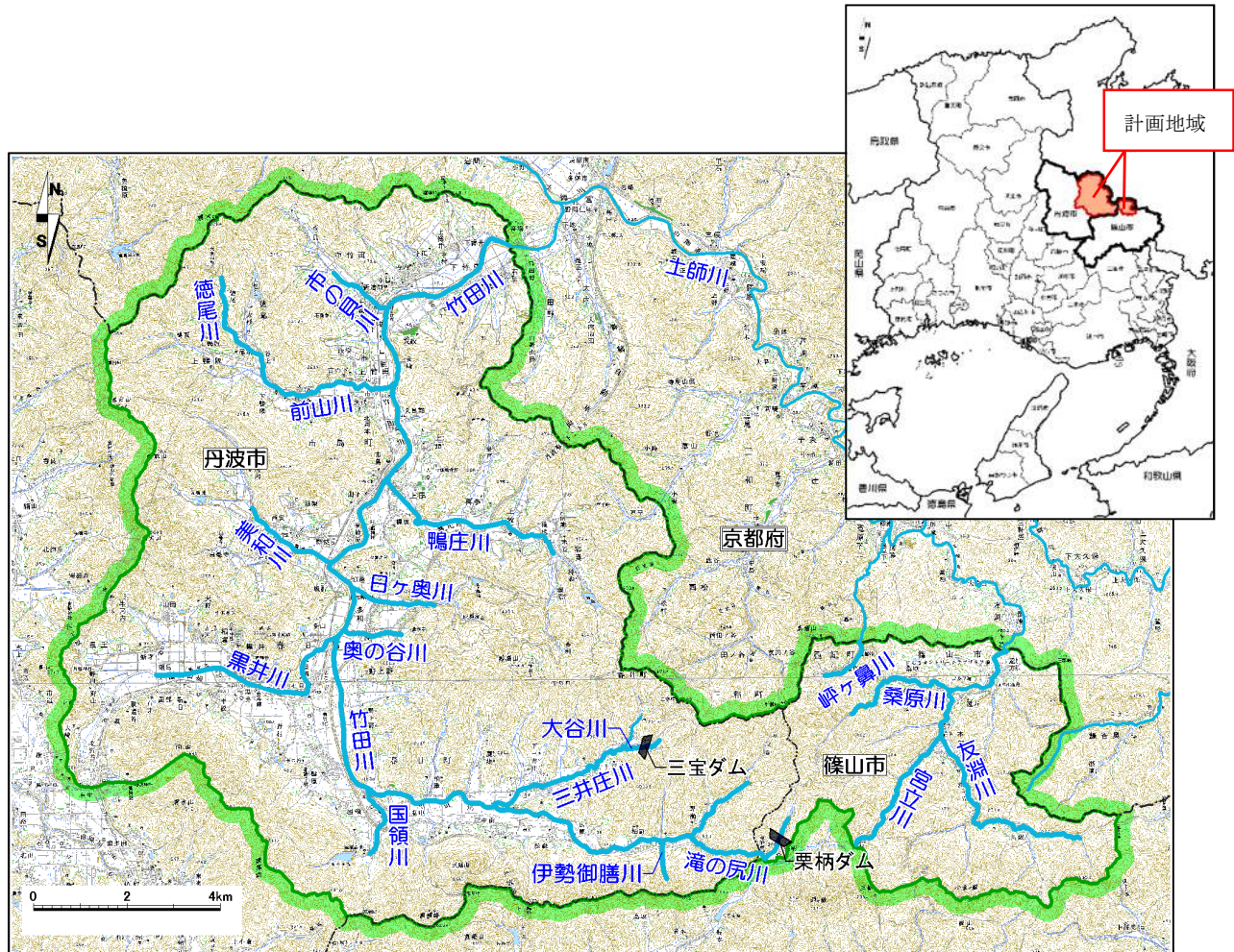
計画地域流域図
