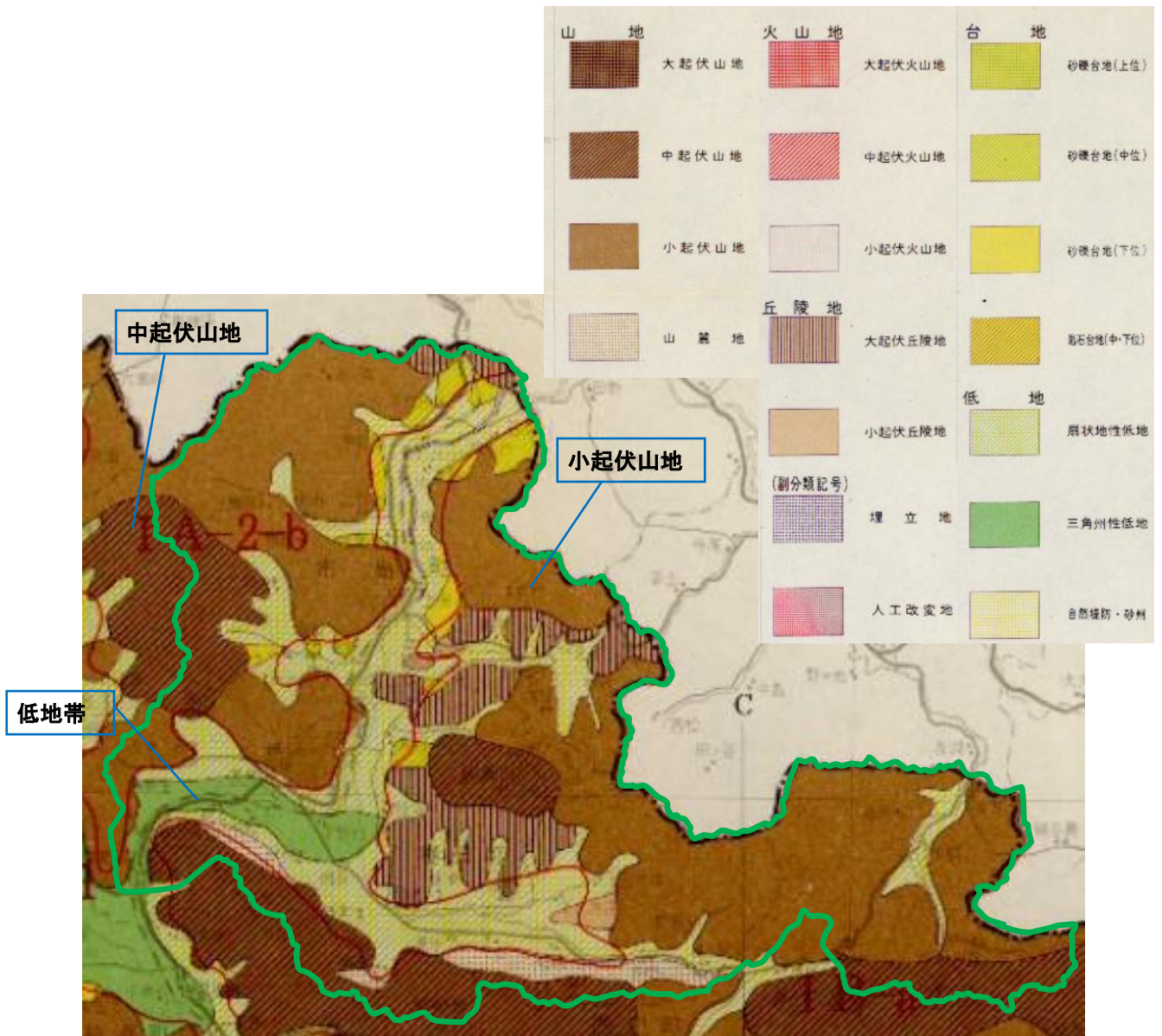
地形分類図
