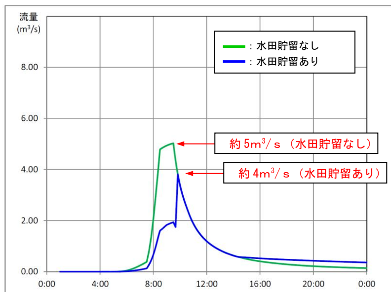
図 10.2.10 水田貯留の効果（水田貯留の有無による水田から樋門付近への流出量の時系列グラフ）
