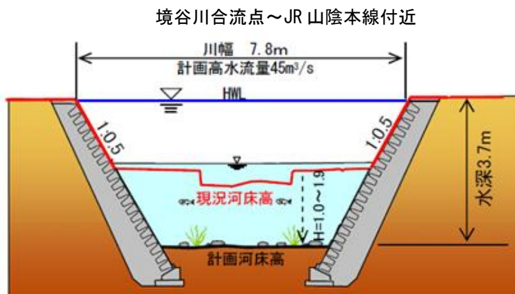
図 1.3.9 香住谷川の改修計画断面の例
