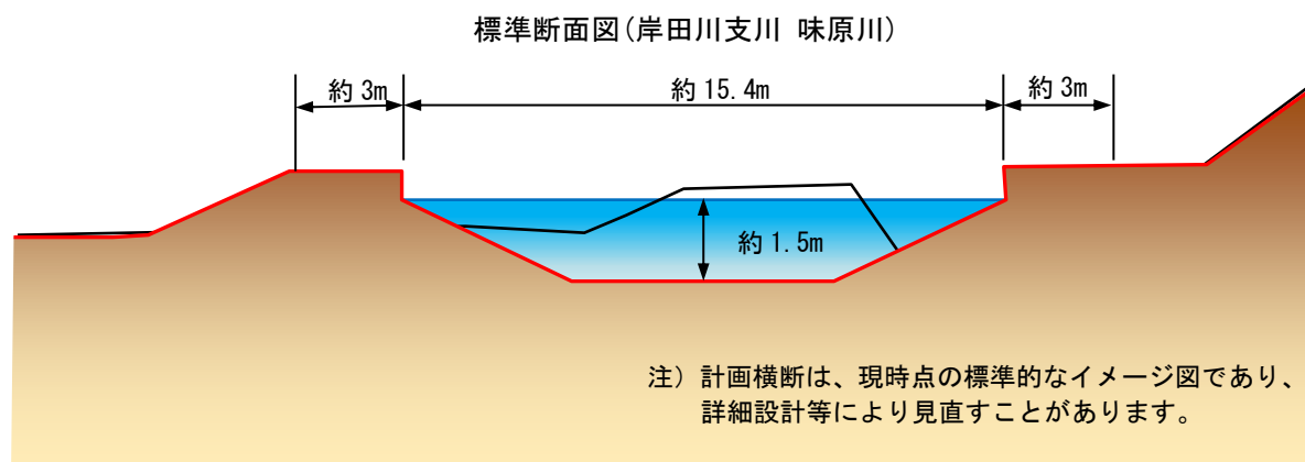
図 1.3.13 岸田川支川 味原川の改修計画断面の例
