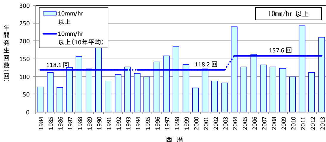
図 1.1.2 但馬地域における近 30 年間の 10mm/hr 以上の降雨の生起回数
