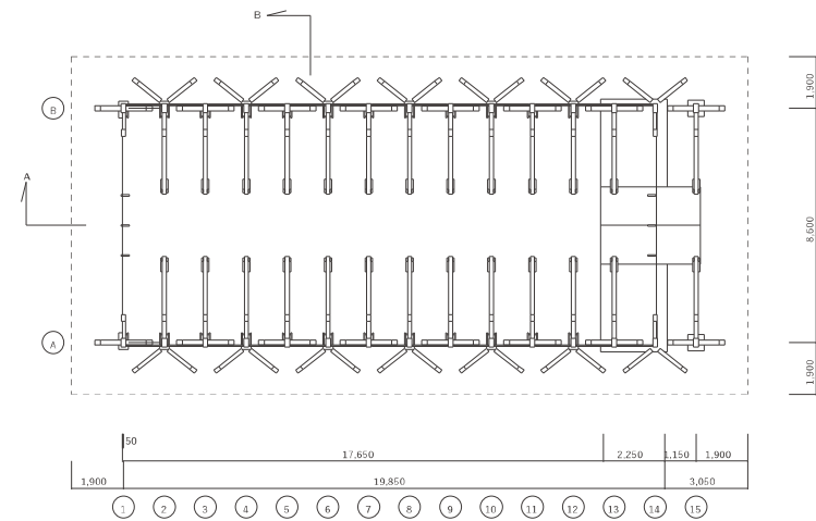
上部平面図 S=1/200
