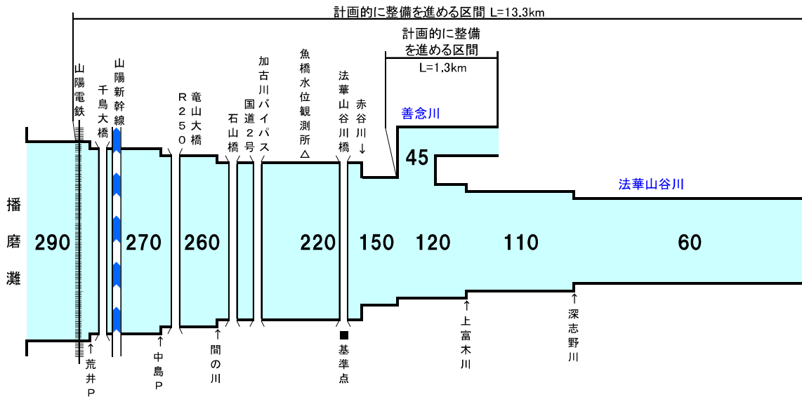
河川整備計画目標流量配分図
