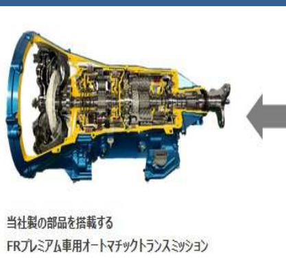
当社製パワートレイン部品
