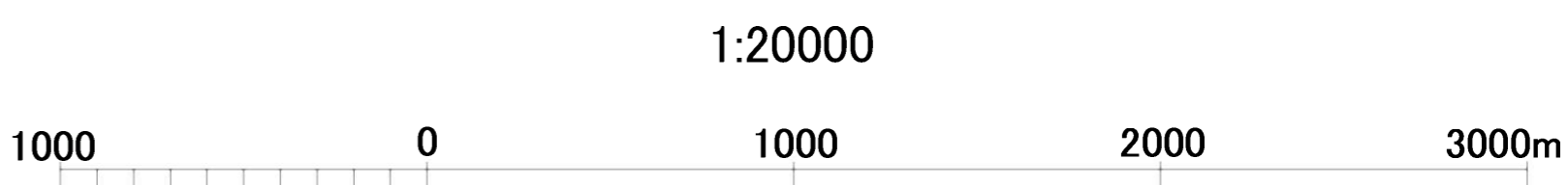
船場川水系 洪水浸水想定区域図 浸水継続時間 総括図(図郭図)
