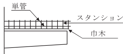
側面図
