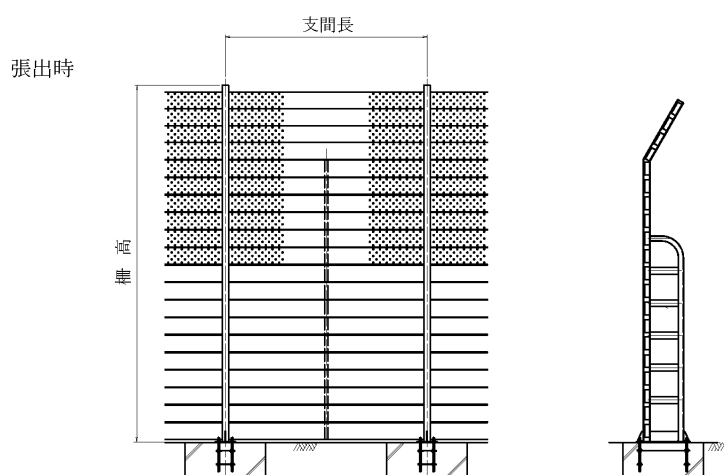
連動型：防雪板全数を同時に張出・収納するタイプ
