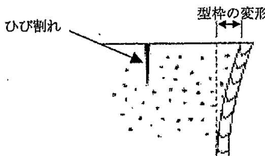
—型枠の変形—
