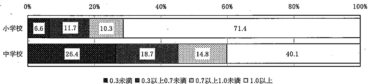
図7 視力の状況
