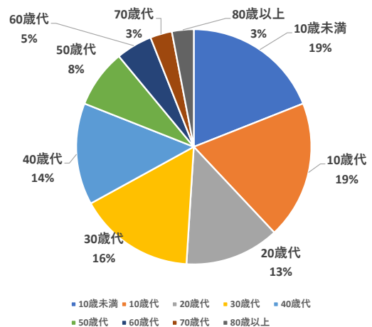
新型コロナウイルス新規感染者の 年齢階級別割合(21週)
