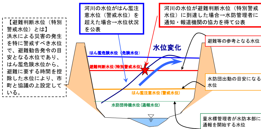
図 8.3.2 特別警戒水位のイメージ図
