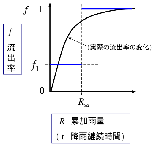
図 - A-3 飽和雨量・流出率 と 累加雨量 の関係
