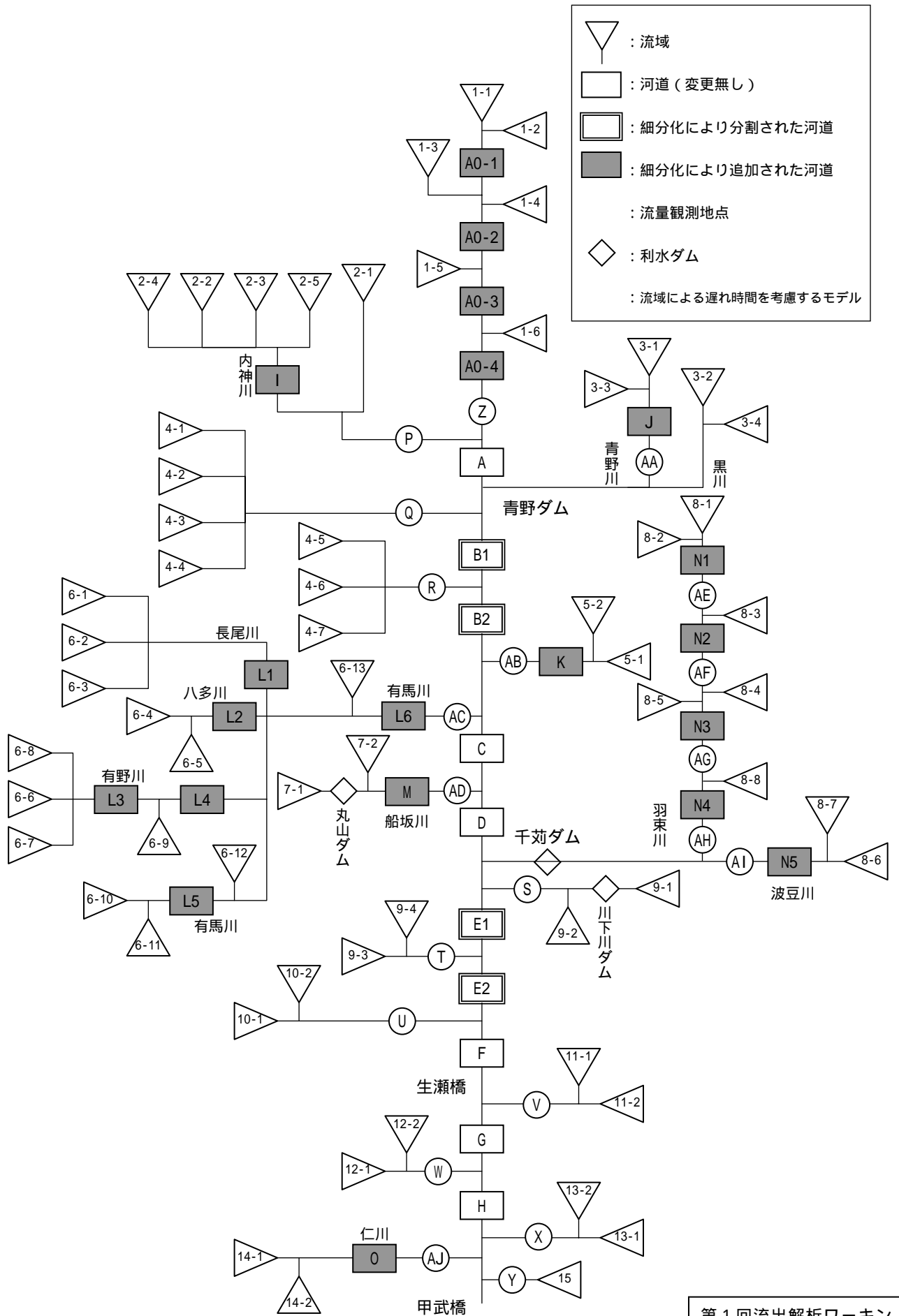
図 6.5.4(2) 武庫川流域流出計算モデル図
