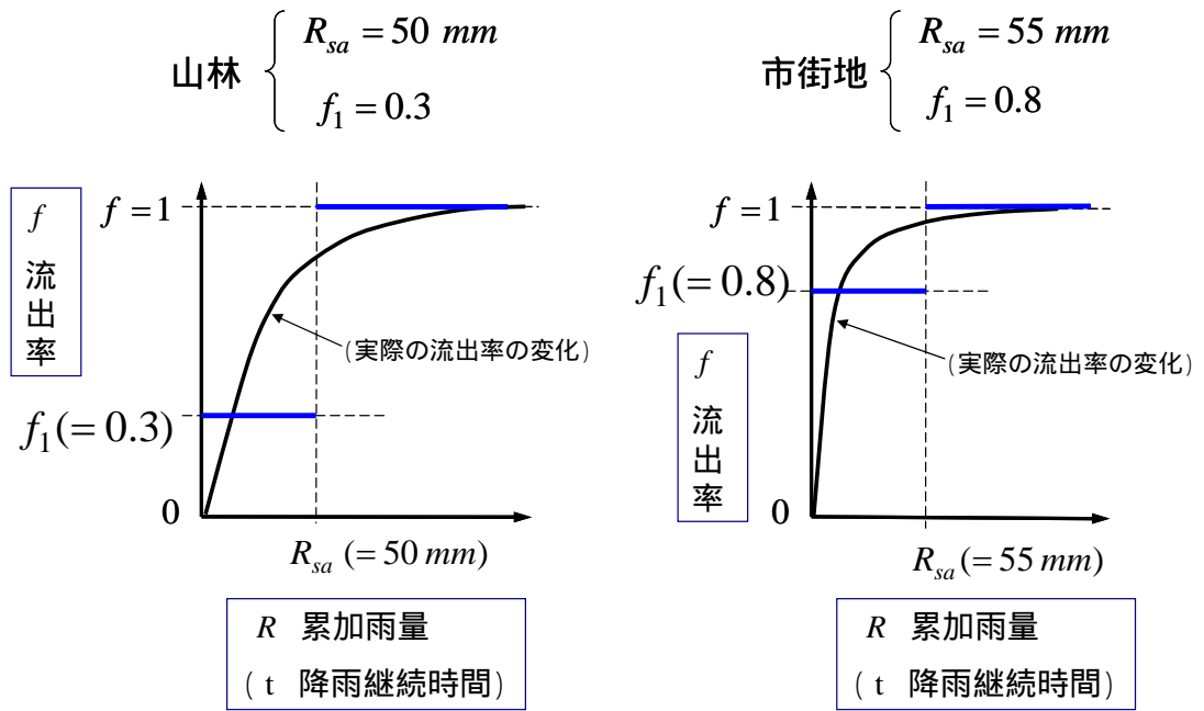
図 - A-4 土地利用別の飽和雨量・流出率と累加雨量の関係
