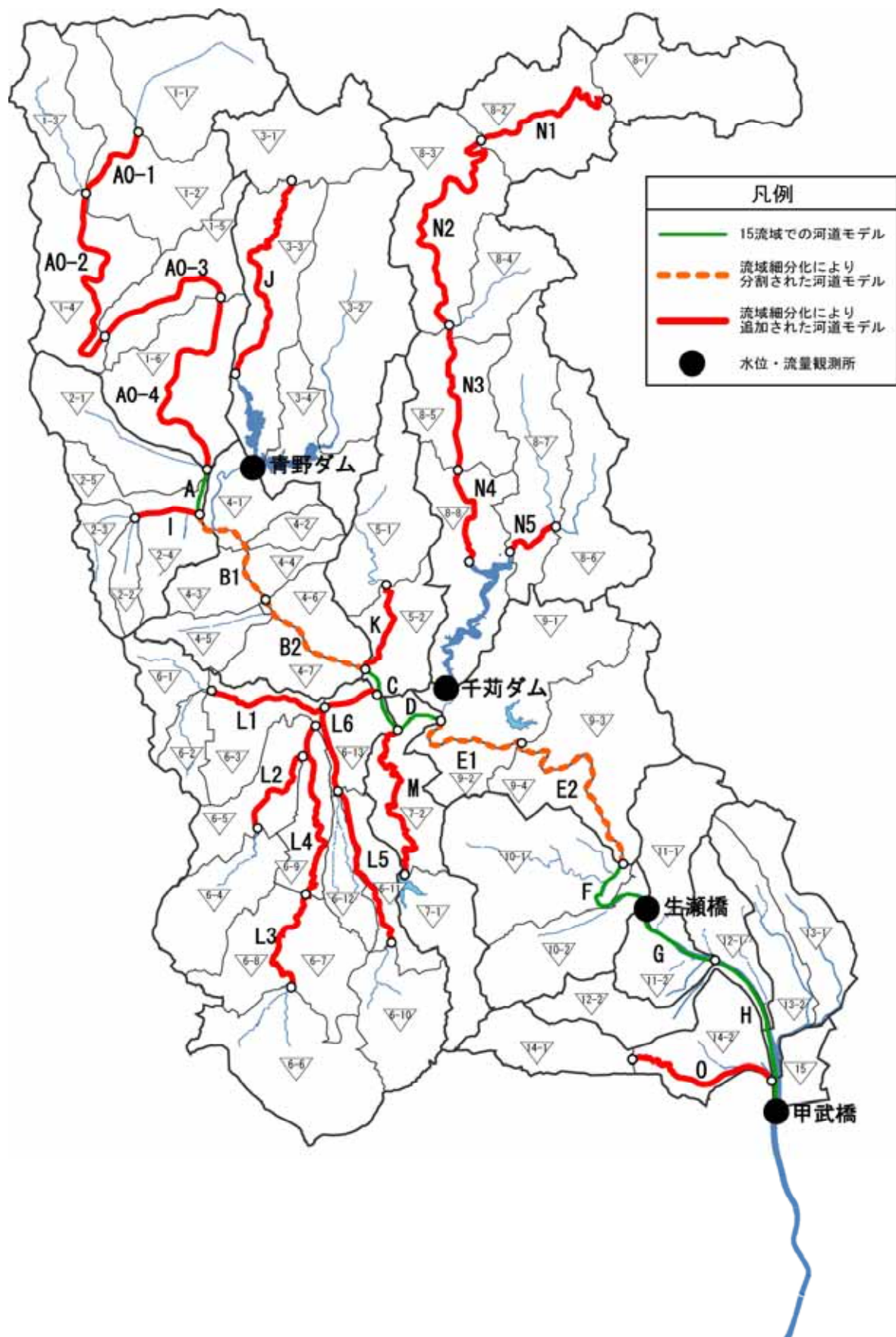
図 6.5.4(1) 武庫川新旧河道モデル比較図
