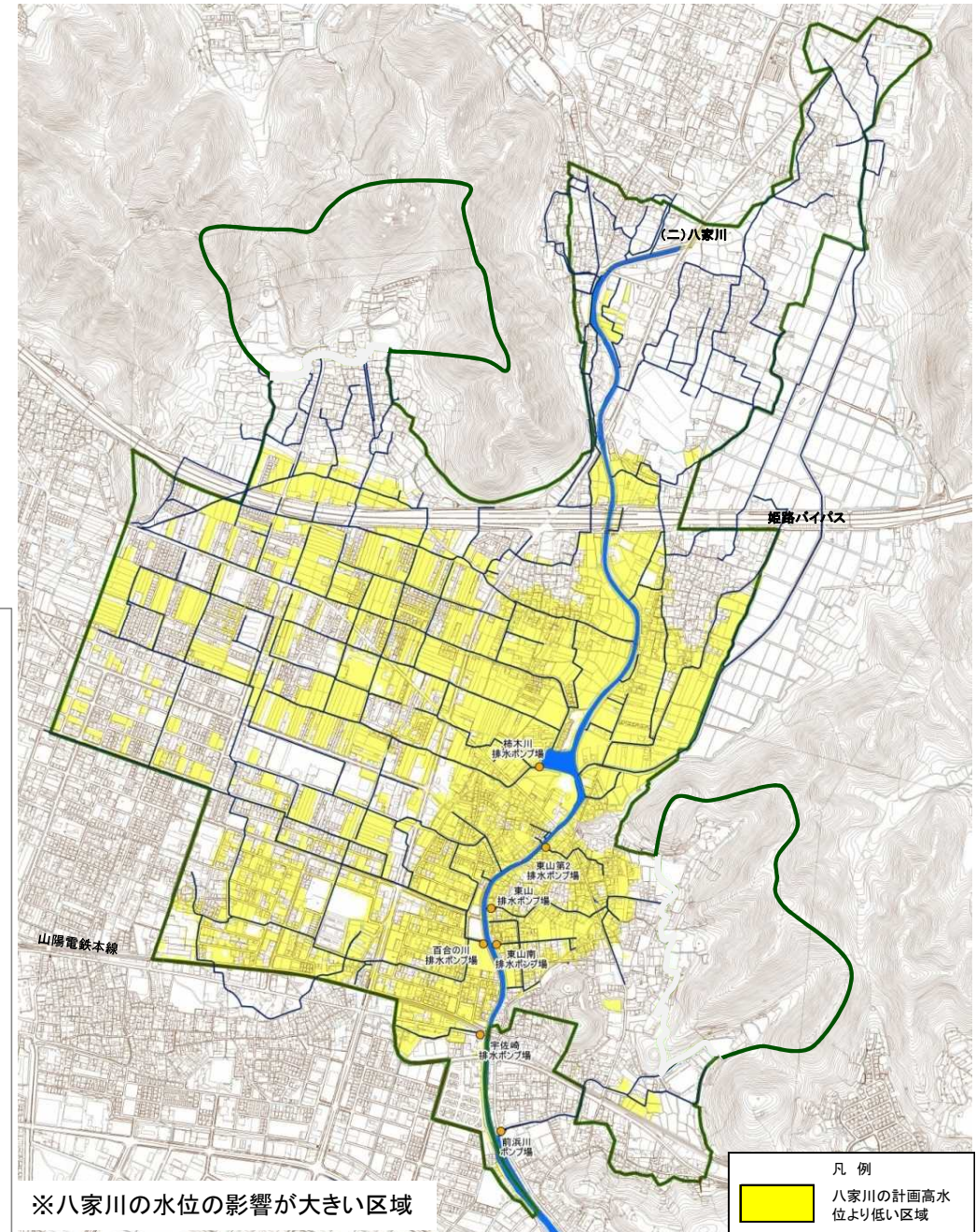
八家川の計画高水位より低い区域
