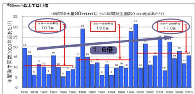
1時間降水量80mm以上の年間発生回数 (1000地点あたり)
