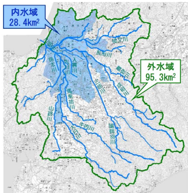
図 46 三原川の内水域
