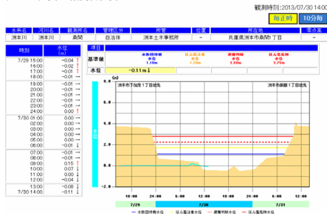
テレメータ水位 桑間(くわま)
