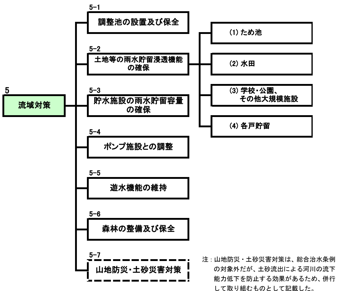
図 28 流域対策の体系
