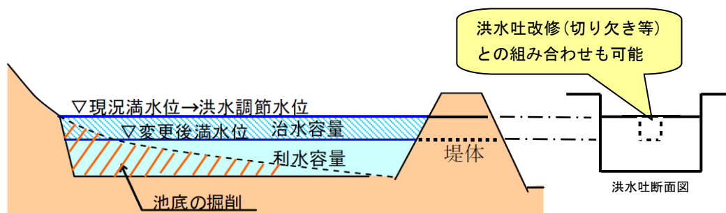
図 29 池底掘削による治水容量の確保イメージ
