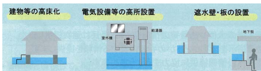
図 43 耐水機能の主な例
