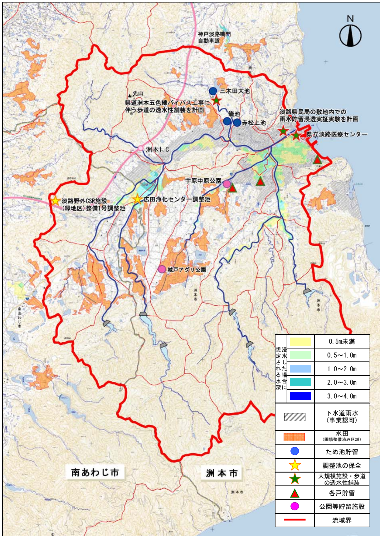
図 49 流域対策モデル地区(洲本川水系)
