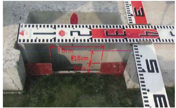
堰板 切り欠き部の寸法 幅 15cm(全体幅の半分程度)×高さ 5cm 製作費 400 円/枚(鉄板錆止め塗装、近隣の鉄工所で作製) (農地・水保全管理支払交付金制度を活用)
